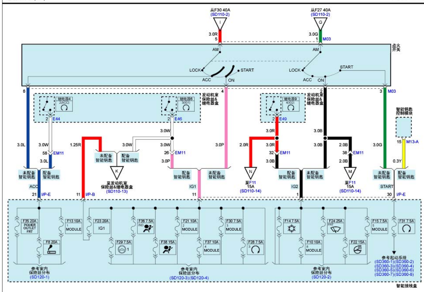
电源分布(15)
